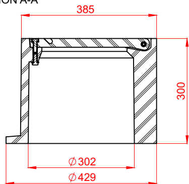
SECCIÓN A-A
